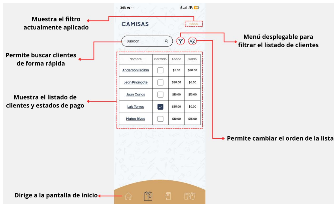
Figura 9 Pantalla de Listado de Camisas
